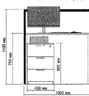
Вид стойки сзади (изнутри).
