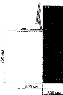
Вид стойки сбоку.
