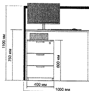
Вид стойки сзади (изнутри).
