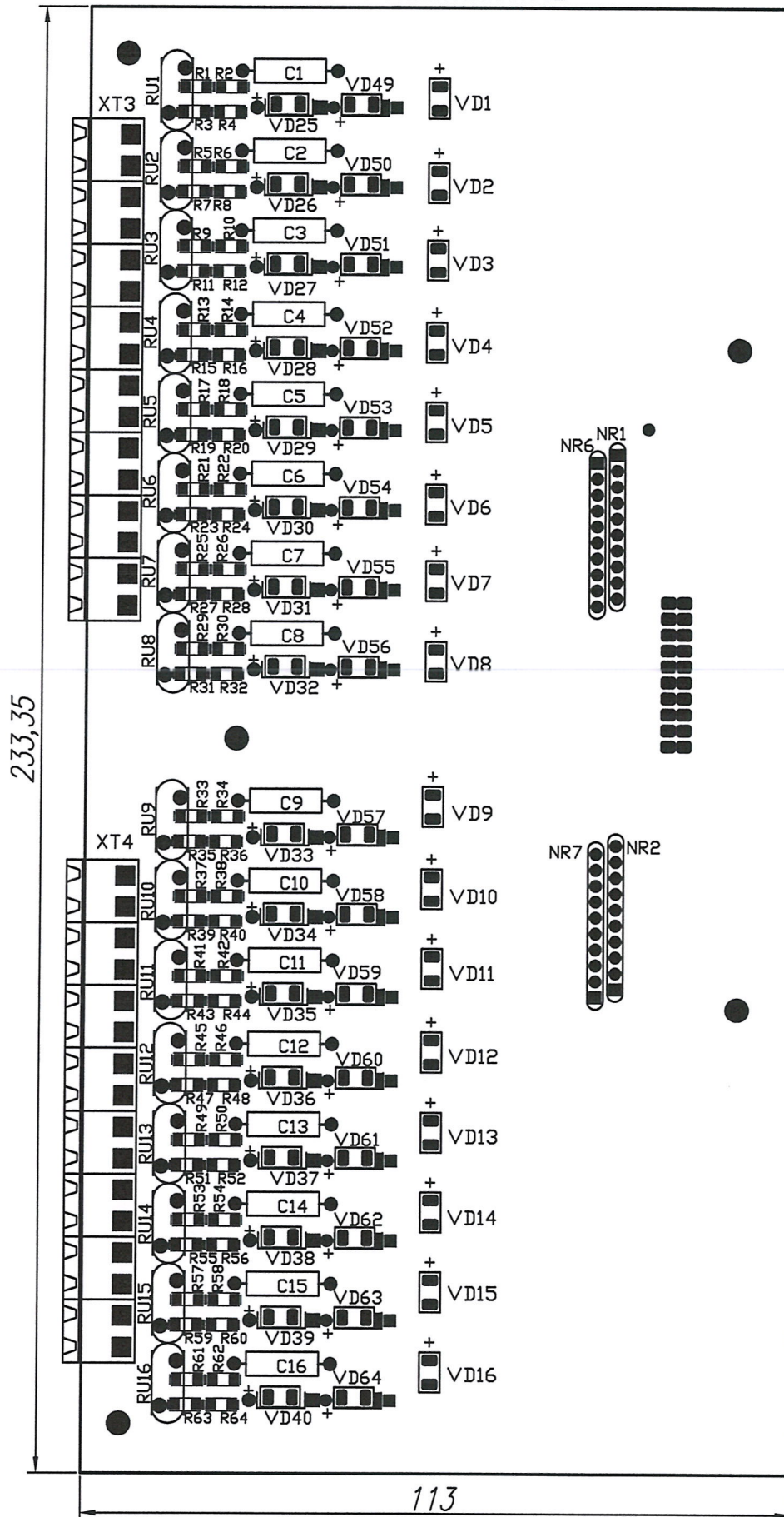
Сборочный чертеж субмодуля MR7_SMS_D16 ПШИЖ 142.21.02.00.002
