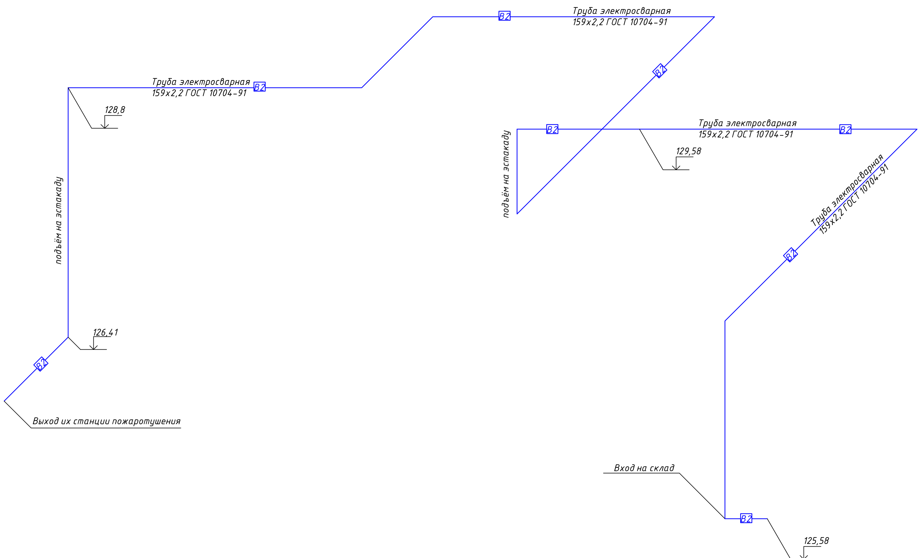
Аксонетрическая схема В2
