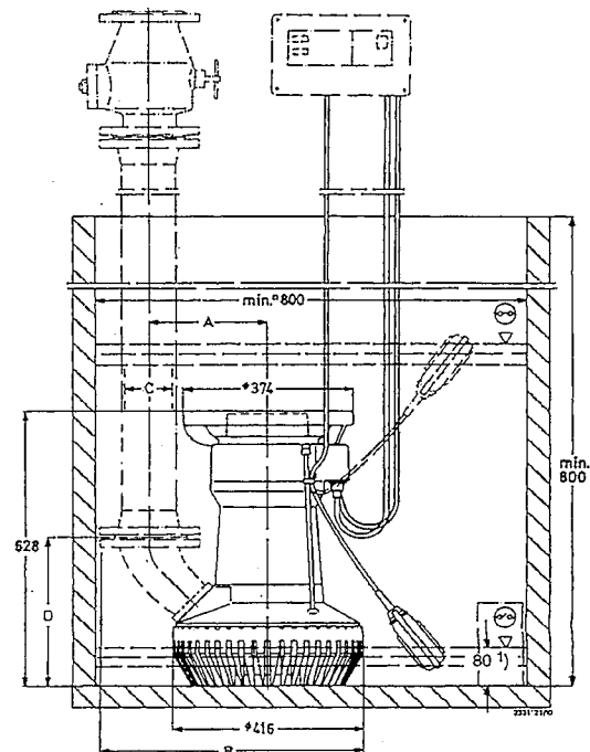
Ama-Drainer 100 SD
