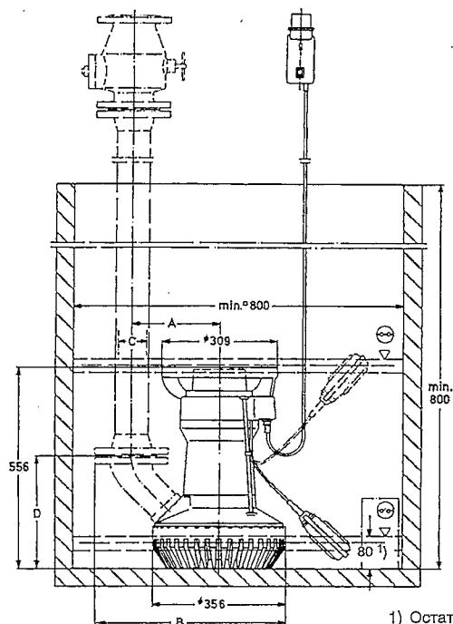
Ama-Drainer 80 SD
