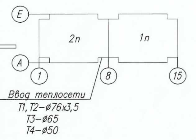
Схема здания
