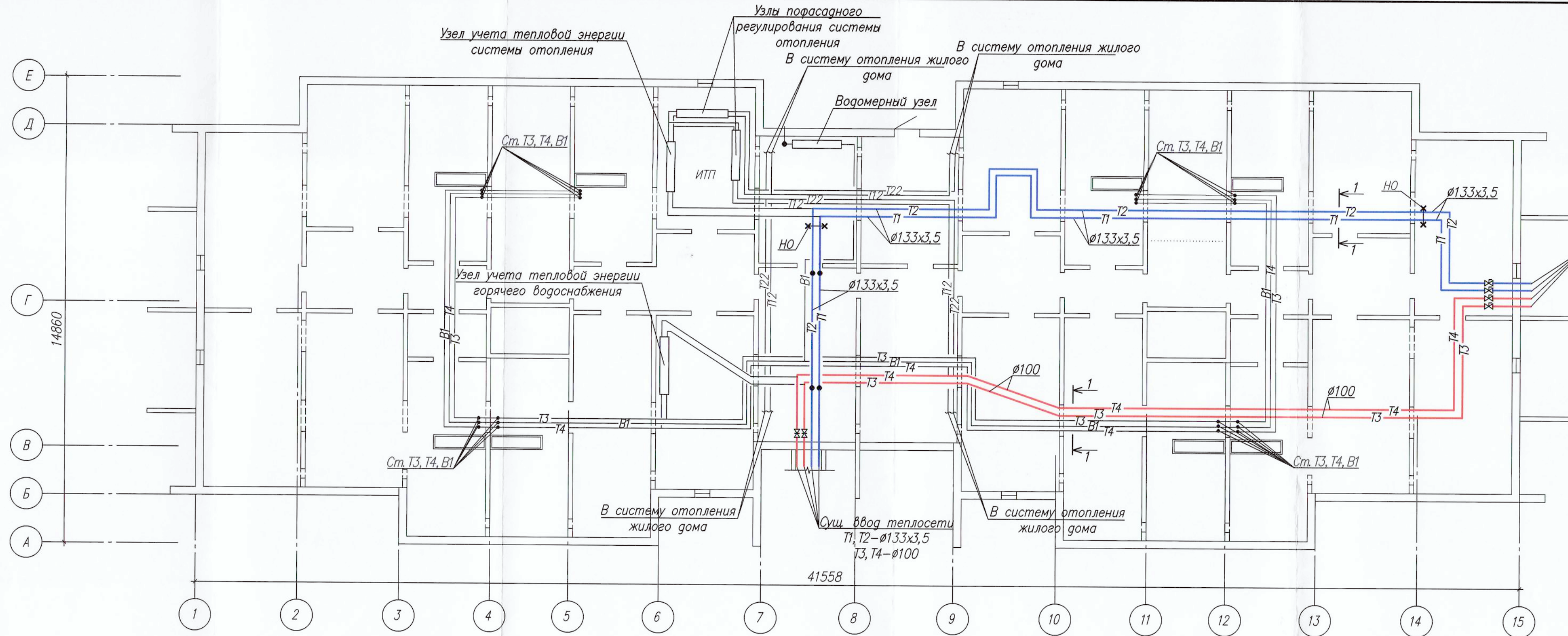
Схема здания
