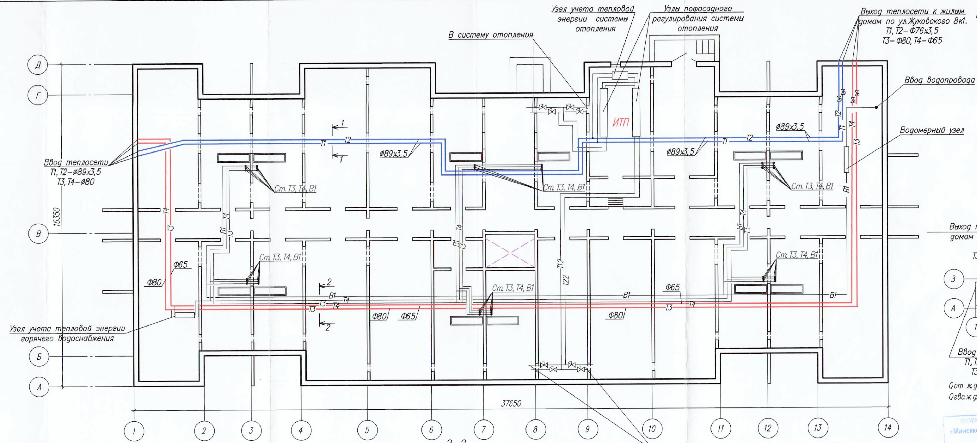
Схема здания
