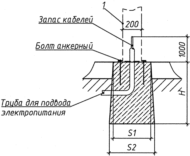
А Фундамент с подводом инженерных коммуникаций
