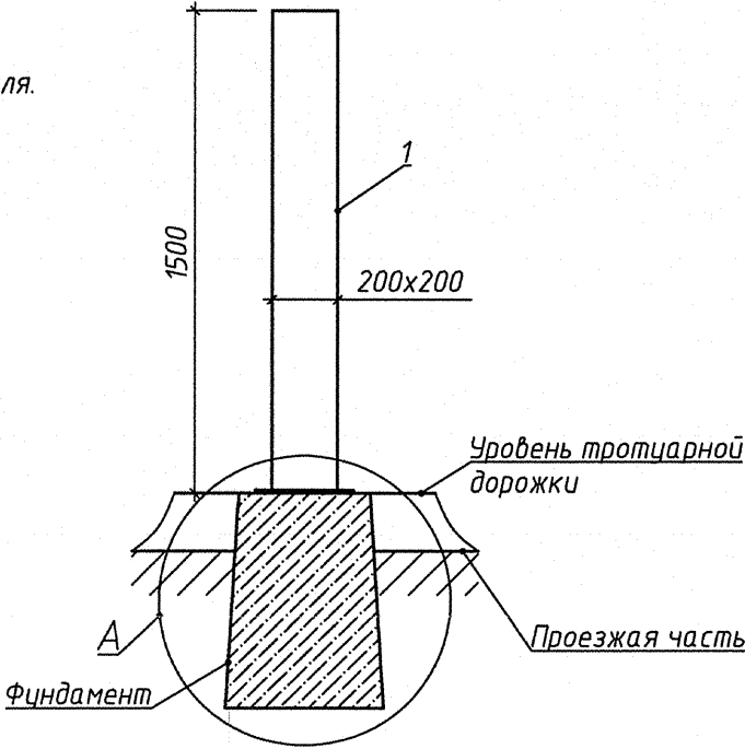
А Фундамент с подводом инженерных коммуникаций
