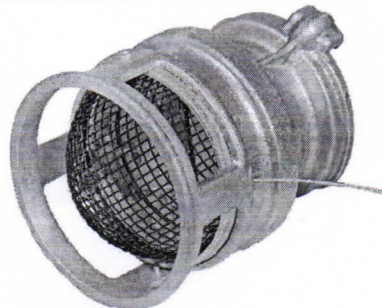
Рисунок. Внешний вид всасывающей пожарной сетки СВ-80
